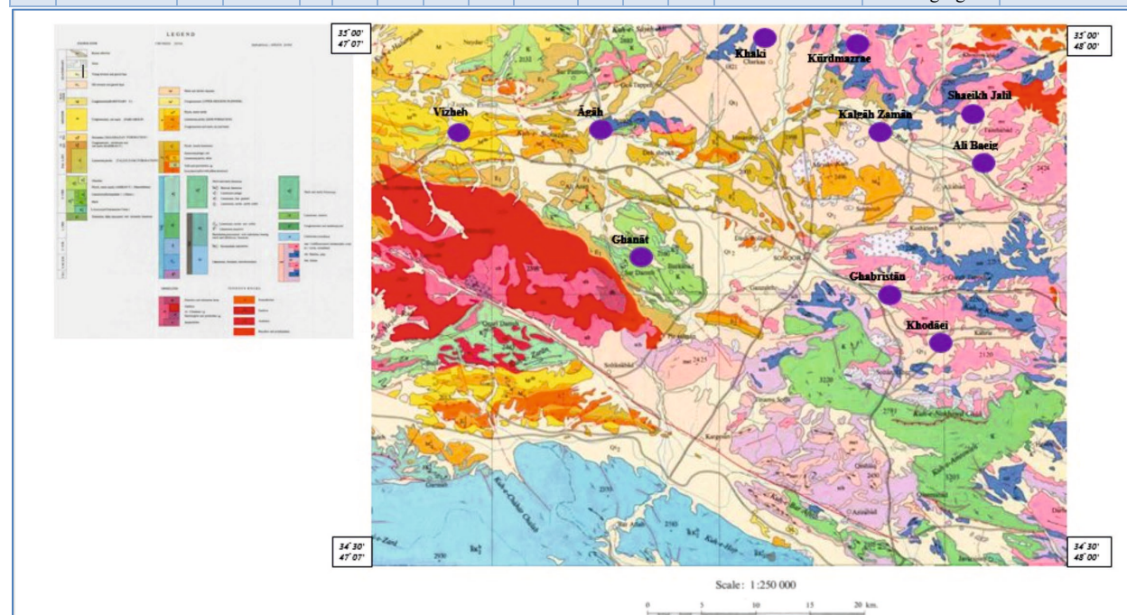
Fig. 3. Geologic Map of Sonqor
